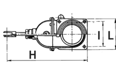
Doppelflanschschieber
