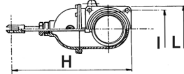
Doppelflanschschieber
