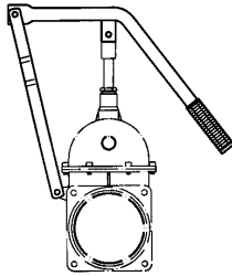
Hebelgarnitur
